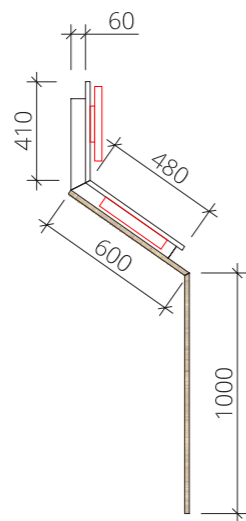
Seitenansicht
