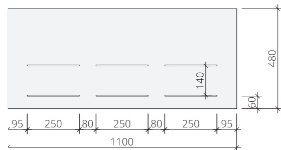
Einlagenhalter
